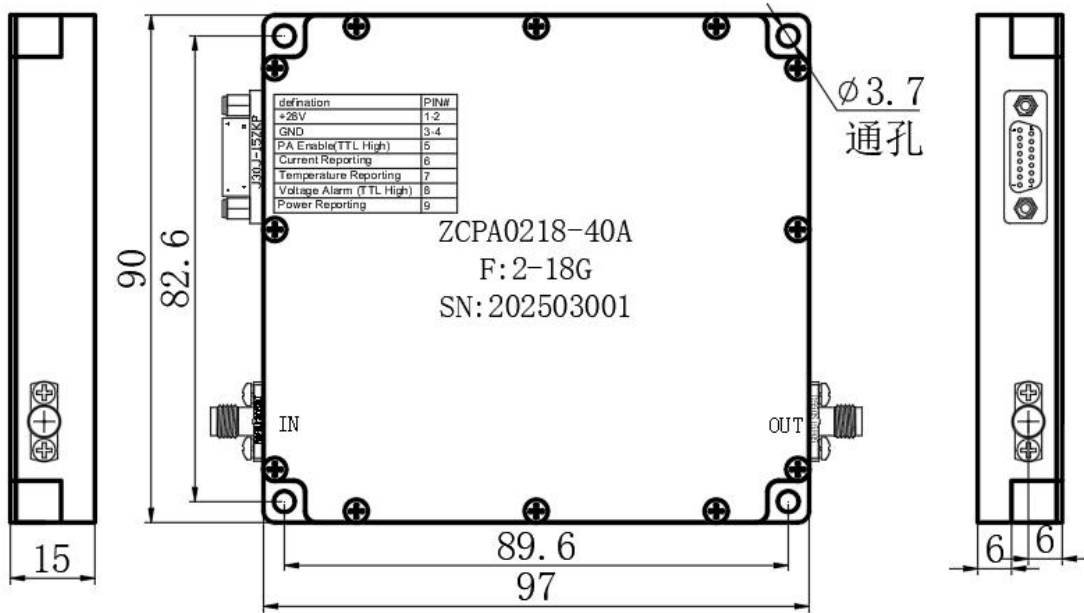
外形尺寸图
