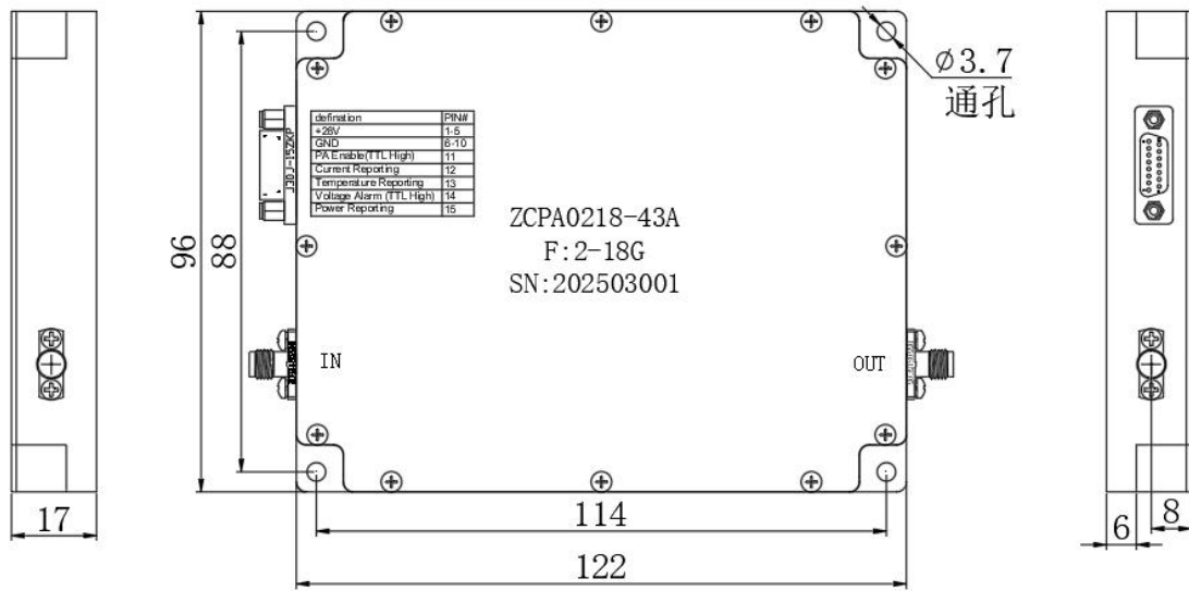
外形尺寸图
