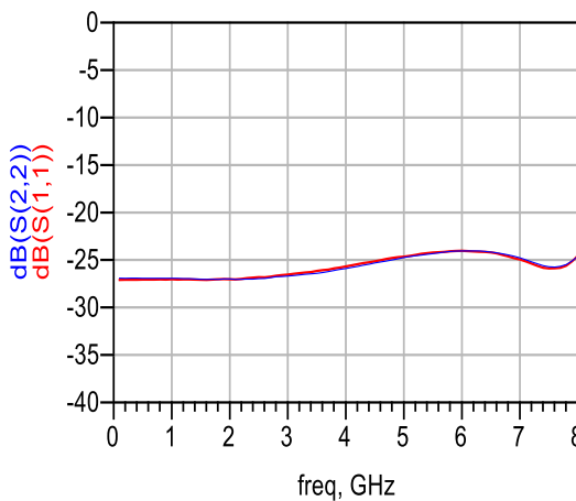
输入输出回波 vs 频率
