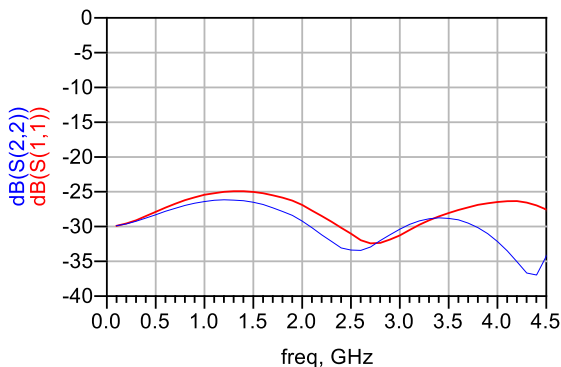
输入输出回波 vs 频率
