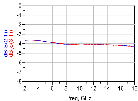
插损 vs 频率
