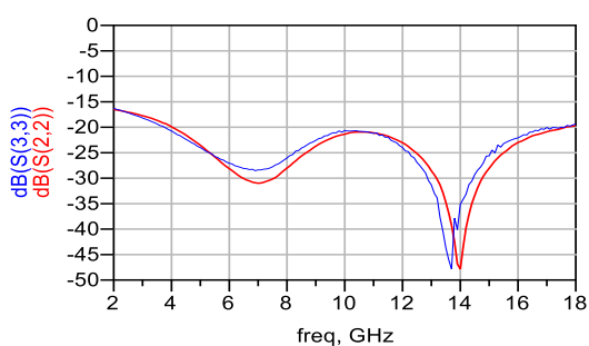
输出回波 vs 频率
