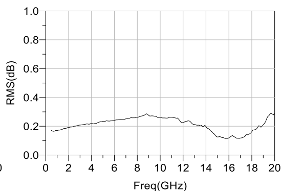
RMS vs 频率
