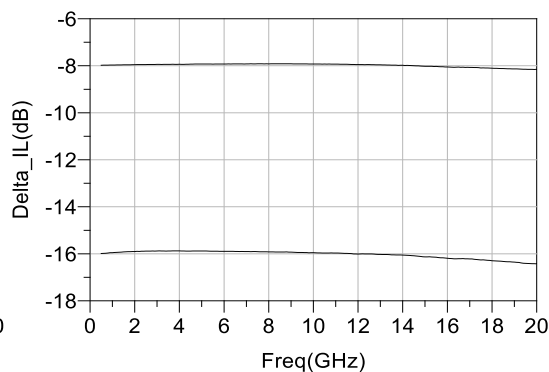
主衰减位 vs 频率
