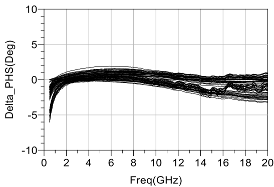
附加移相 vs 频率
